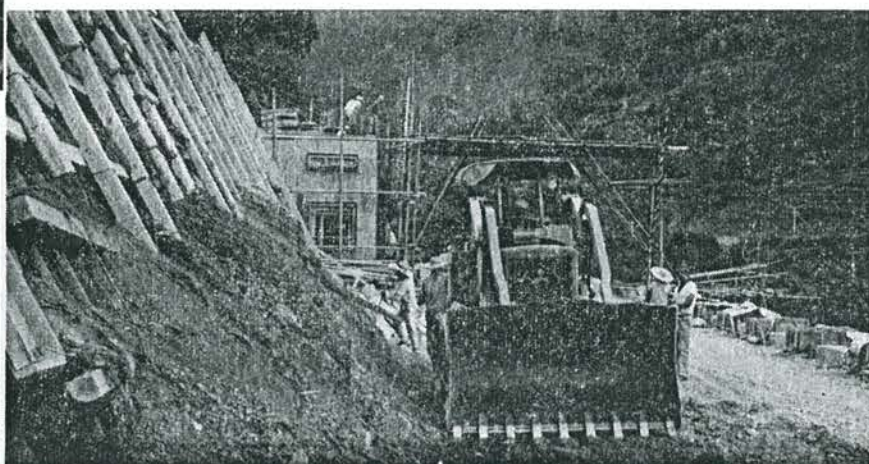
左・発電所のそばでは、国道改良工事もおこなわれています。 上・建設中の発電所、上からみたところ
